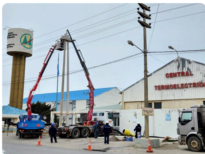
IZAJE EN CENTRAL TERMOELÉCTRICA
